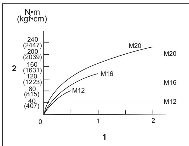
1. Tiempo de apriete (segundo) 2. Par de apriete
