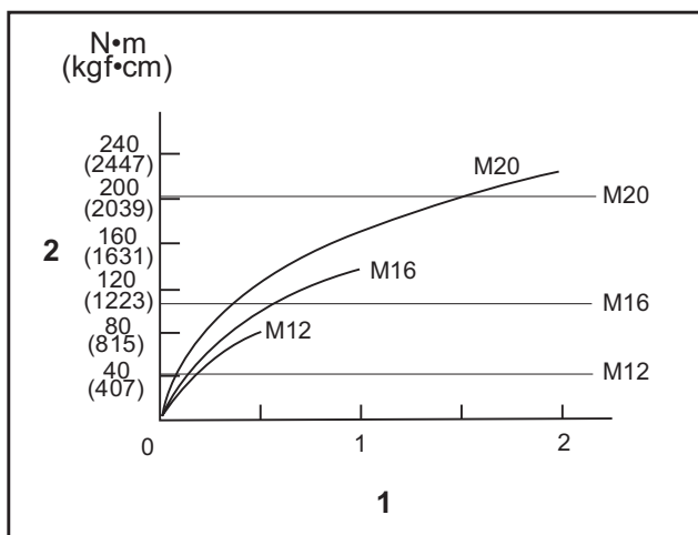
1. Tilspændingstid (sekunder) 2. Tilspændingsmoment
