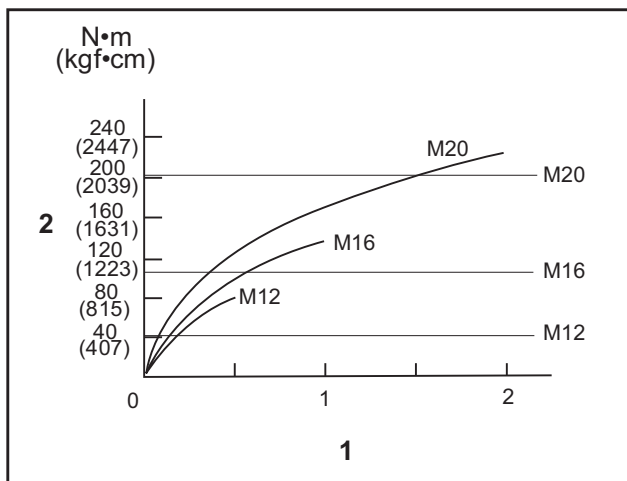
1. Aandraaitijd (seconden) 2. Aandraaimoment
