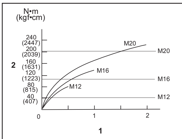
1. Anzugszeit (Sekunden) 2. Anzugsmoment
