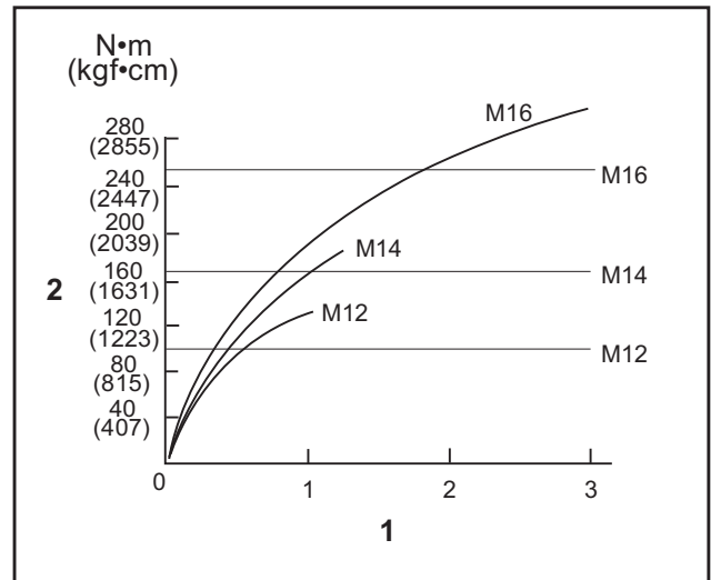
1. Tempo di serraggio (secondi) 2. Coppia di serraggio
