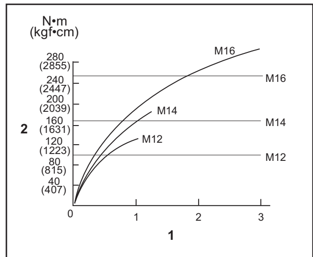
1. Tiempo de apriete (segundo) 2. Par de apriete
