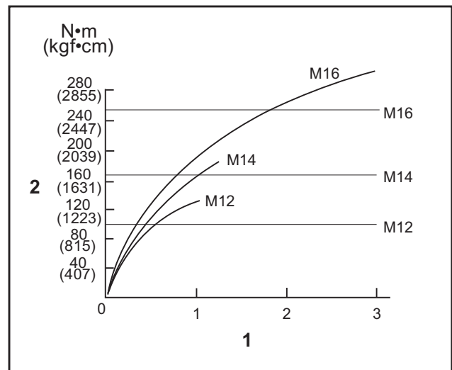
1. Aandraaitijd (seconden) 2. Aandraaimoment
