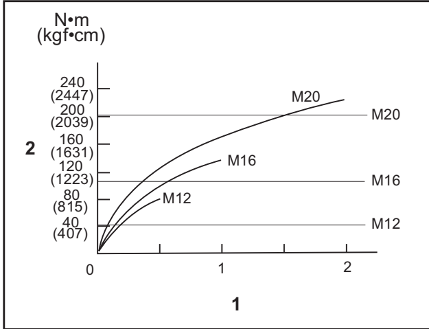
1. Sıkma süresi (saniye) 2. Sıkma torku
