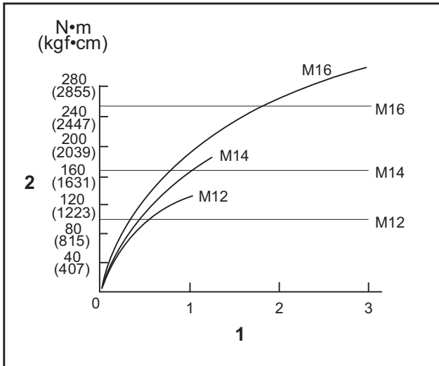
1. Sıkma süresi (saniye) 2. Sıkma torku
