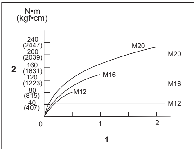
1. Tempo di serraggio (secondi) 2. Coppia di serraggio
